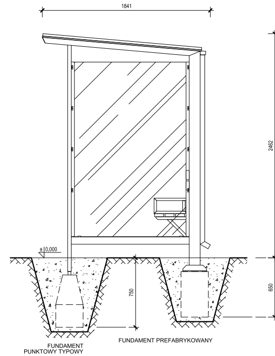
ELEWACJA PRAWA
