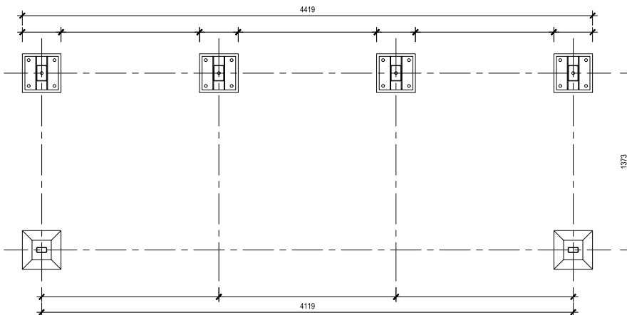
RZUT FUNDAMENTÓW 1:25
